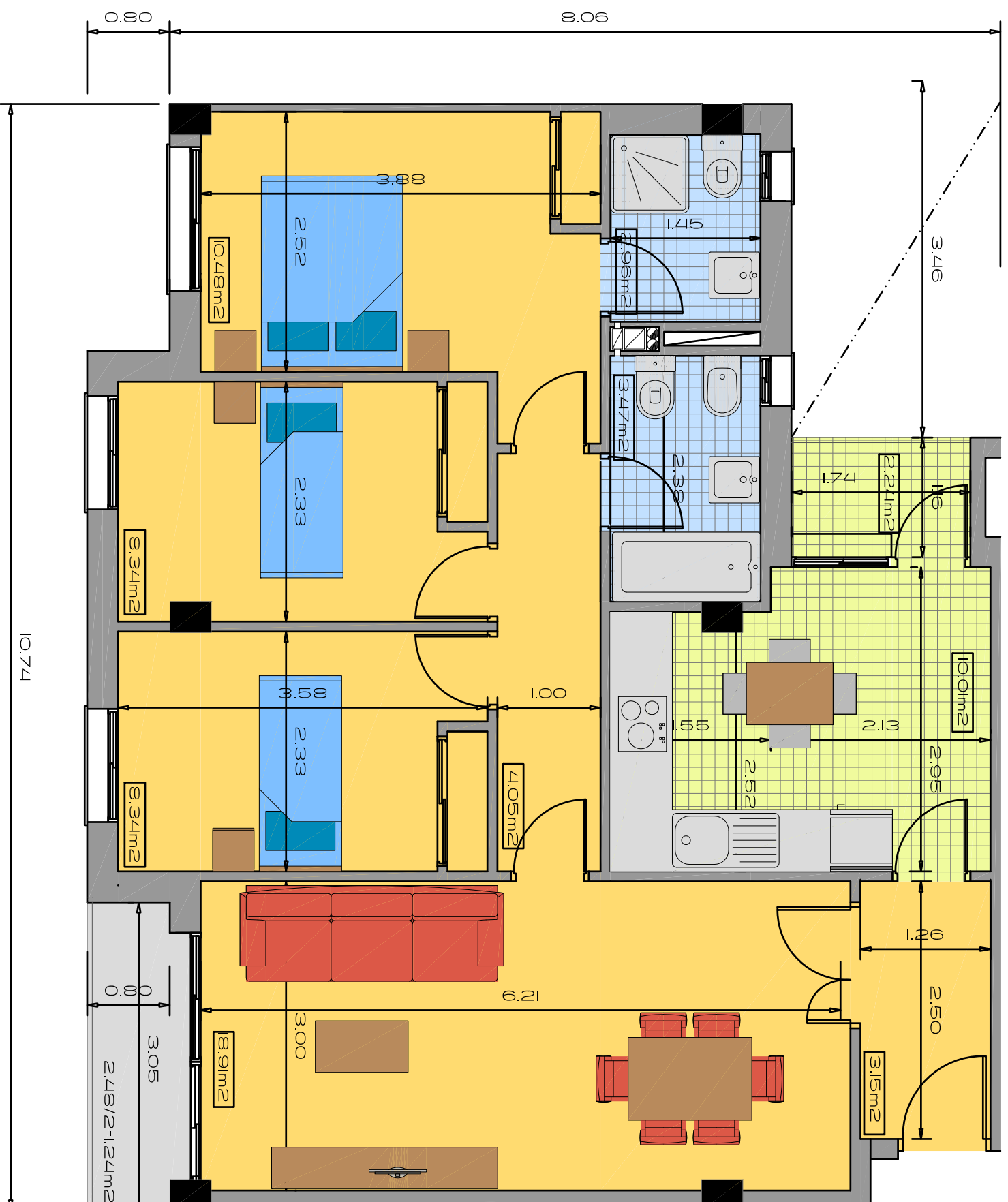
VIVIENDA TIPO - 3 DORMITORIOS ESCALA 1:50
